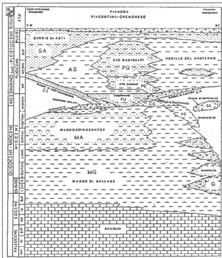
Figura 6: Rapporti litostратigrafici nell'area centrale padana (Dondi, 1985)
