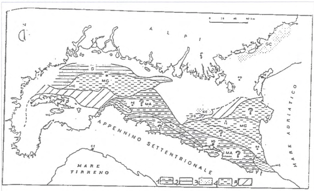
Figura 2: Bacino padano: carta delle litofacies nel Langhiano. 1: Marnoso-arenacea (MA); 2: Gonfolite (G); 3: Glauconie di Cavanella (GC); 4: Marne di Gallare (MG); 5: aree emerse (da Dondi, 1985).
